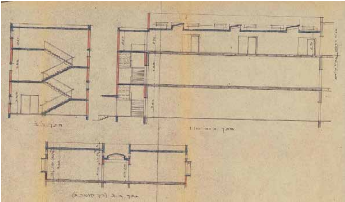
חתך המבנה עם תוספת הקומה
