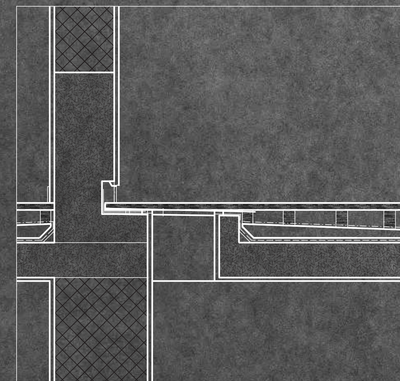
פרט תאורה טבעית 1:10
